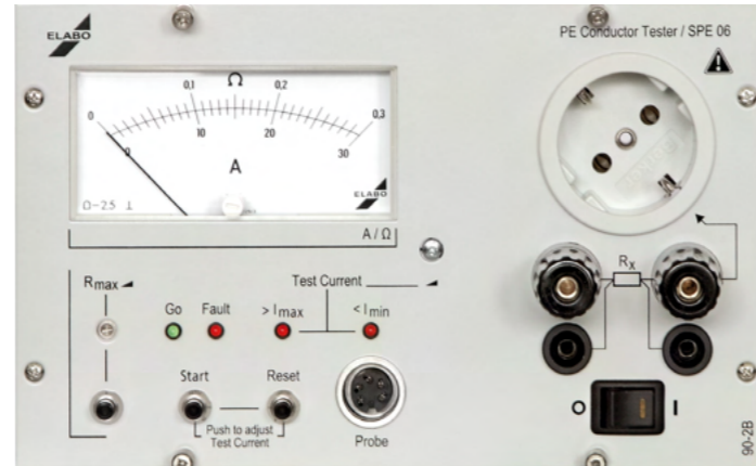
Frontansicht 90-2B
