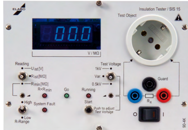
Frontansicht 90-4K
