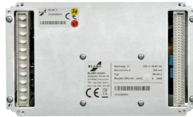
Rückansicht 90-4K
