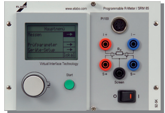
Frontansicht 92-5K
